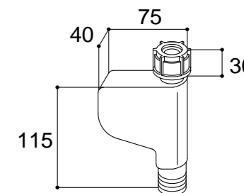
給水電磁弁 詳細
