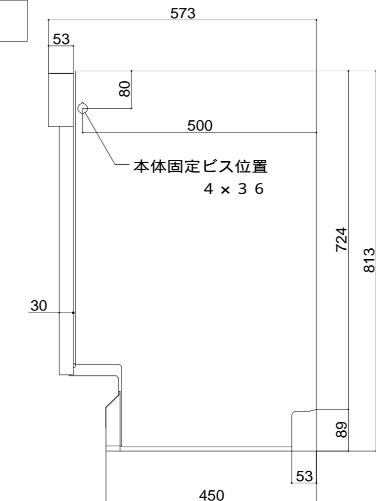
側面図
