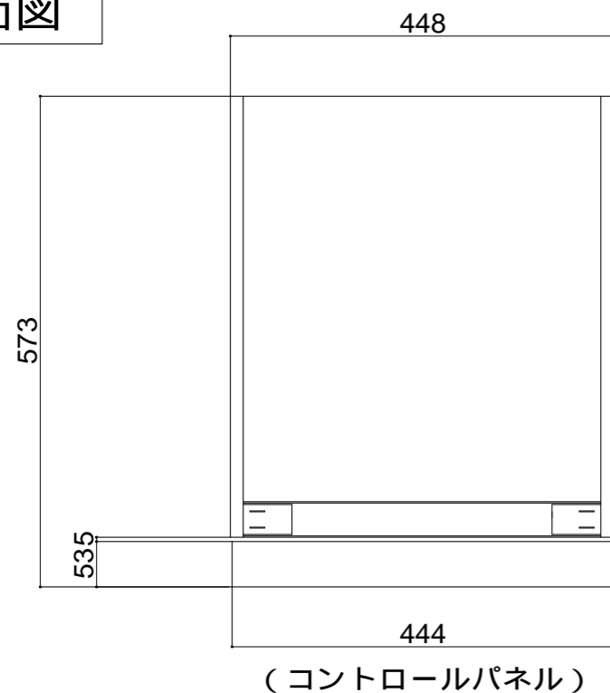
正面図
